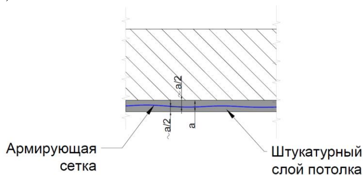
Рис. 15. Армированный штукатурный слой в местах стыка разных материалов и плит перекрытия
